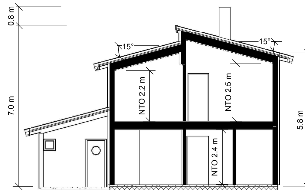
Snitt A-A
