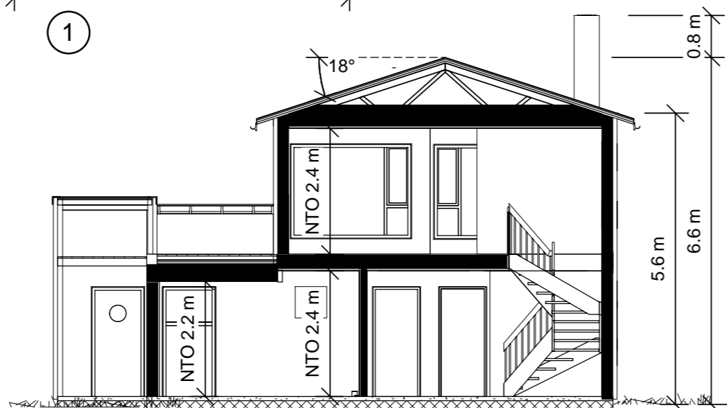
SNITT A-A
