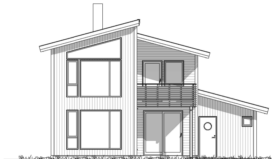
FASADE 1
